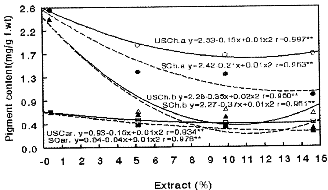
شكل (٤٦): تأثير التركيزات المختلفة لمستخلص نبات الرطريط من المواقع الملحية (S) وغير الملحية (US) على محتوى صبغيات البناء الضوئي (كلورفيل ا، ب والكاروتينات Ch.a, Ch.b, and Car. على التوالي) في أوراق نبات السدر، بالإضافة الى علاقات الارتباط بينهما ممثلة بمنحنيات ومعادلات الانحدار.
