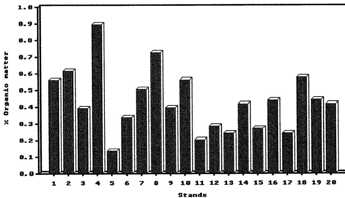
شكل (١٠): التغيرات في النسب المئوية لسعة إحتفاظ التربة بالماء والمادة العضوية بتربة المواقع المختلفة المختارة في منطقة الدراسة.
