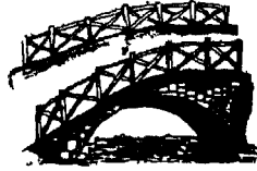
قَنْطَرَةٌ
