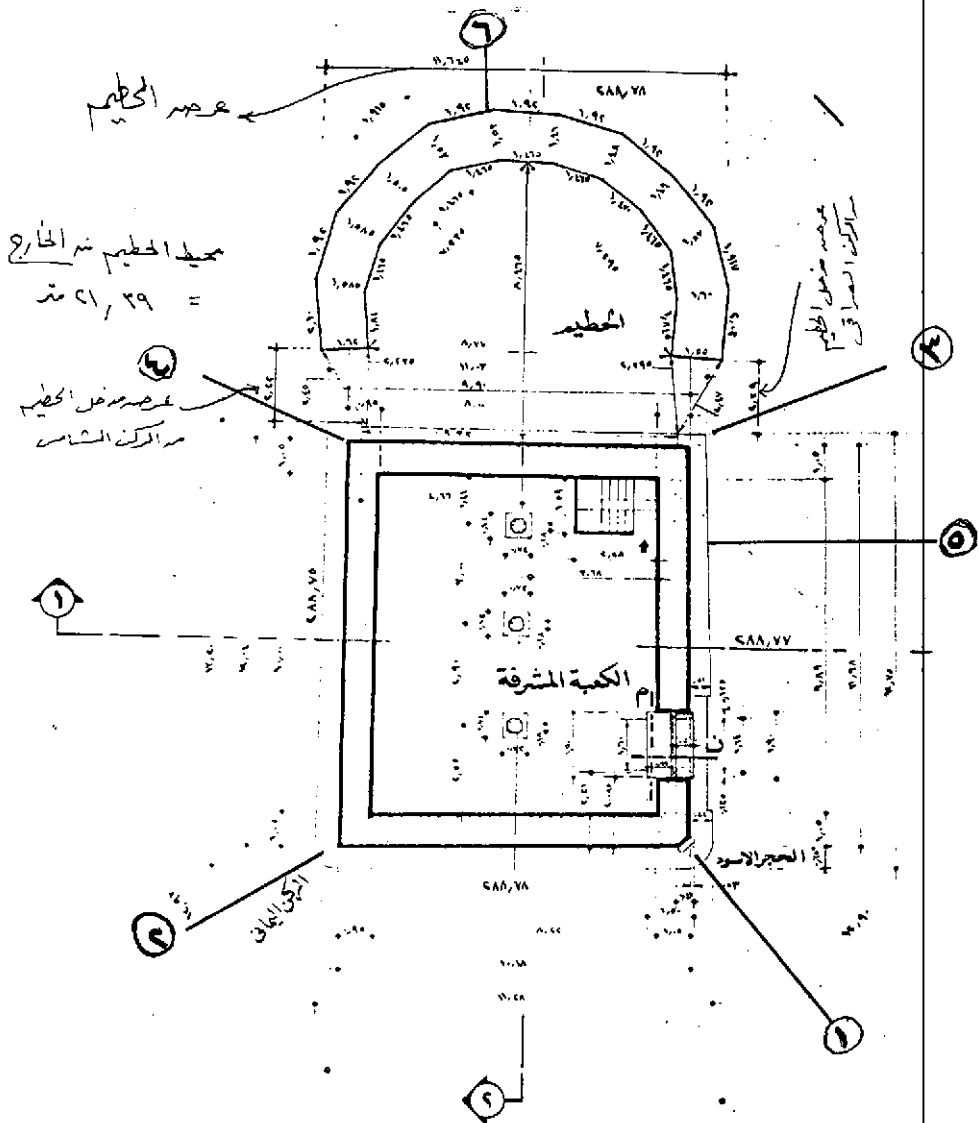
مسقط أفقي للكعبة المشرفة الرئاسة العامة لشؤون المسجد الحرام والمسجد النبوي
