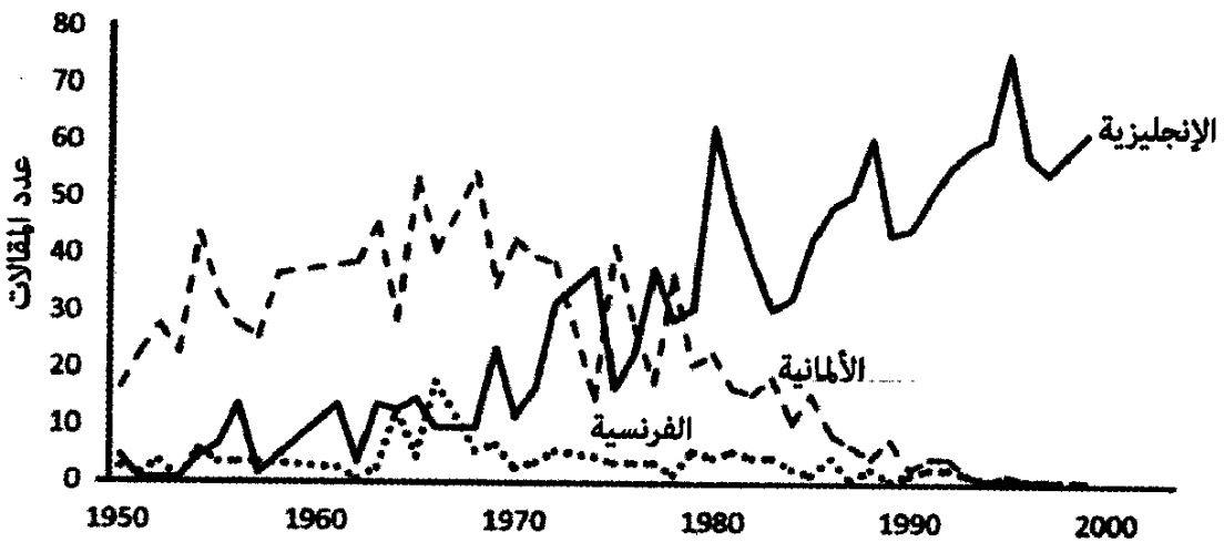
الشكل (3 - 5) عدد المقالات المنشورة في السنة بالألمانية والفرنسية والإنجليزية في مجلة Geologische Rundschau , 1952 - 2000. غيرت المجلة اسمها إلى المجلة الدولية لعلوم طبقات الأرض International Journal of Earth Science في العام 1997.
