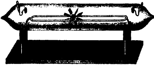
أنابيب كروكس: أشعة الكاثود تضيء ماسة، وتعكس ظلاً للصليب مالطي، وتحرك دولا ب تجديف صغيراً
