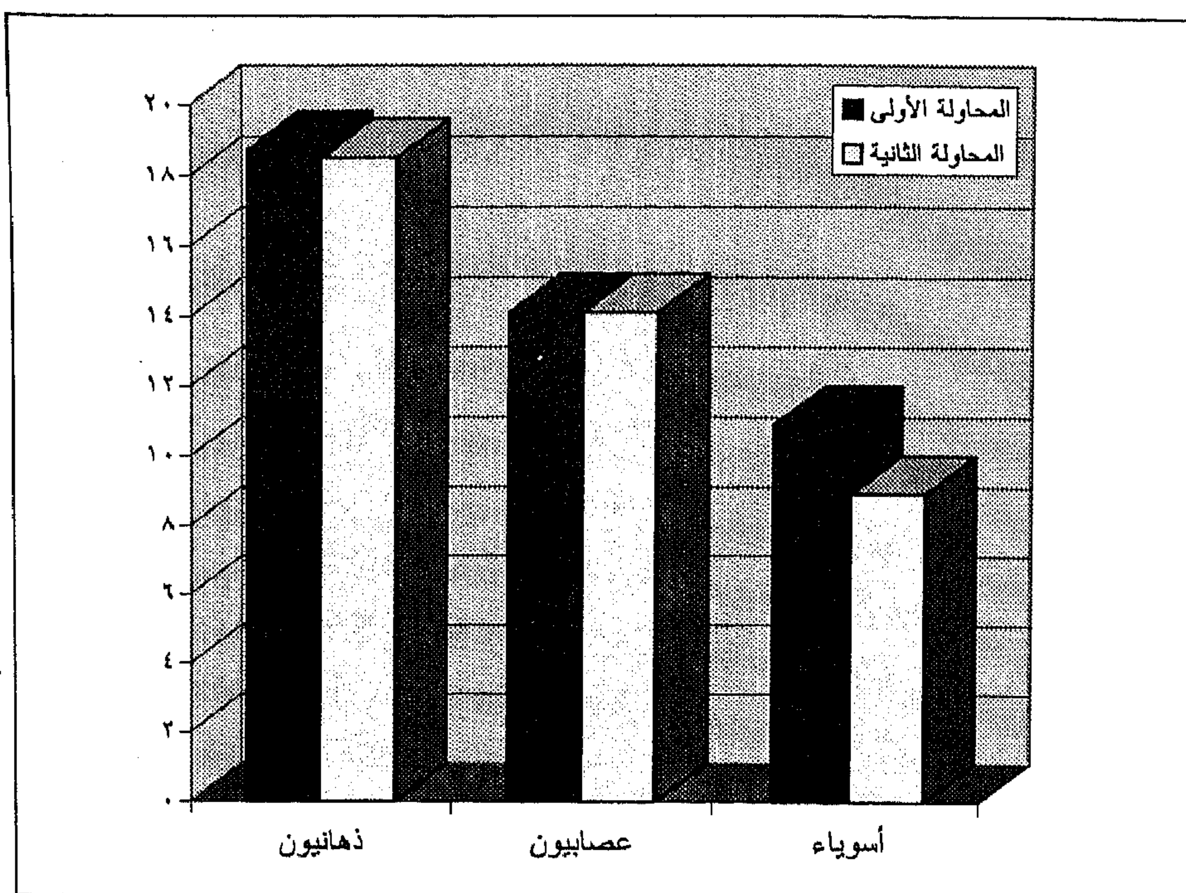
شكل (٣٢) : متوسط الأثر اللاحق لبريمة أرشميدس لدى ثلاث مجموعات من الأسوياء والعصائبيين والذهانيين
