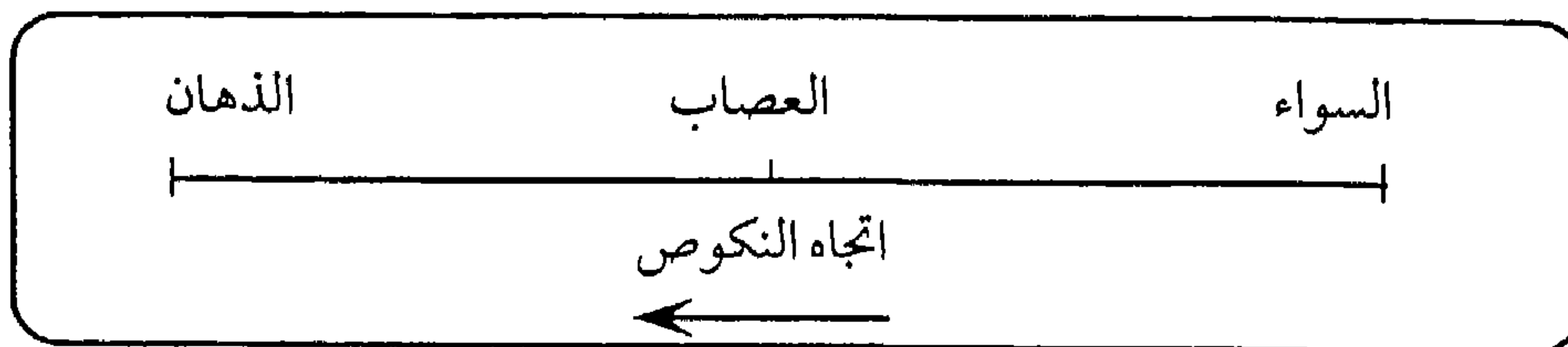
شكل (٨) : تمثيل أحادي البعد للسواء والعصاب والذهان
