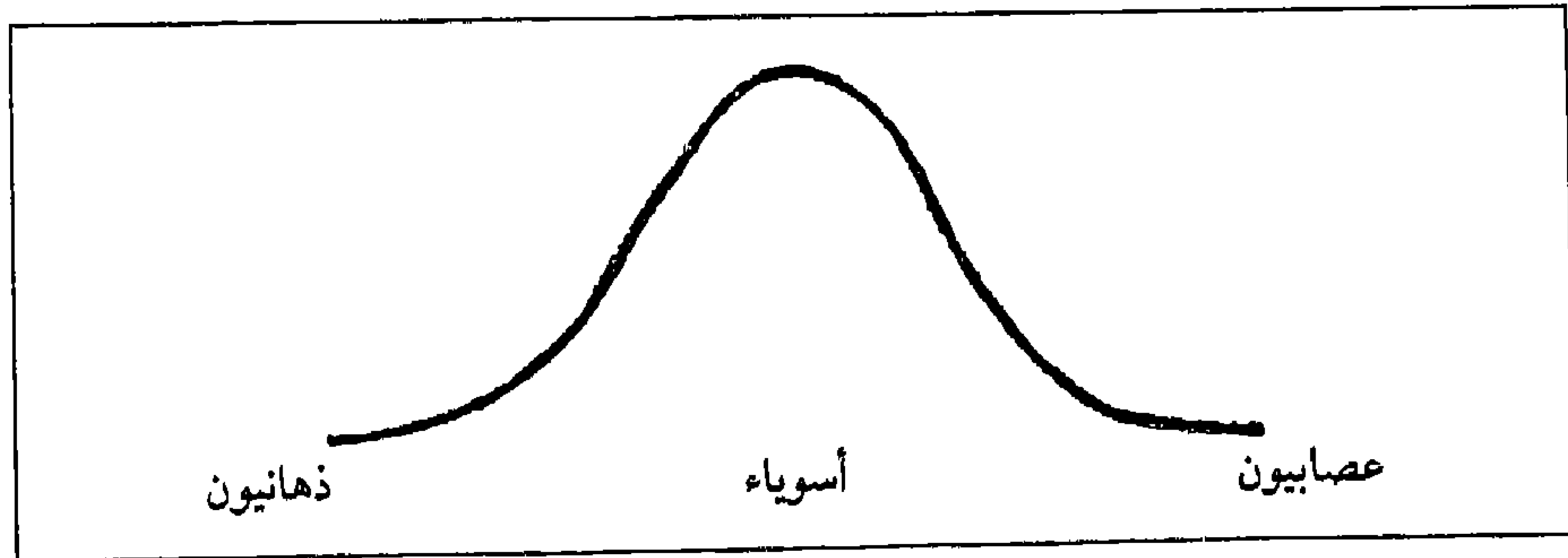
شكل (٧) : توزع الأسوياء والعصابيين والذهانيين على منحنى اعتدالي واحد .
