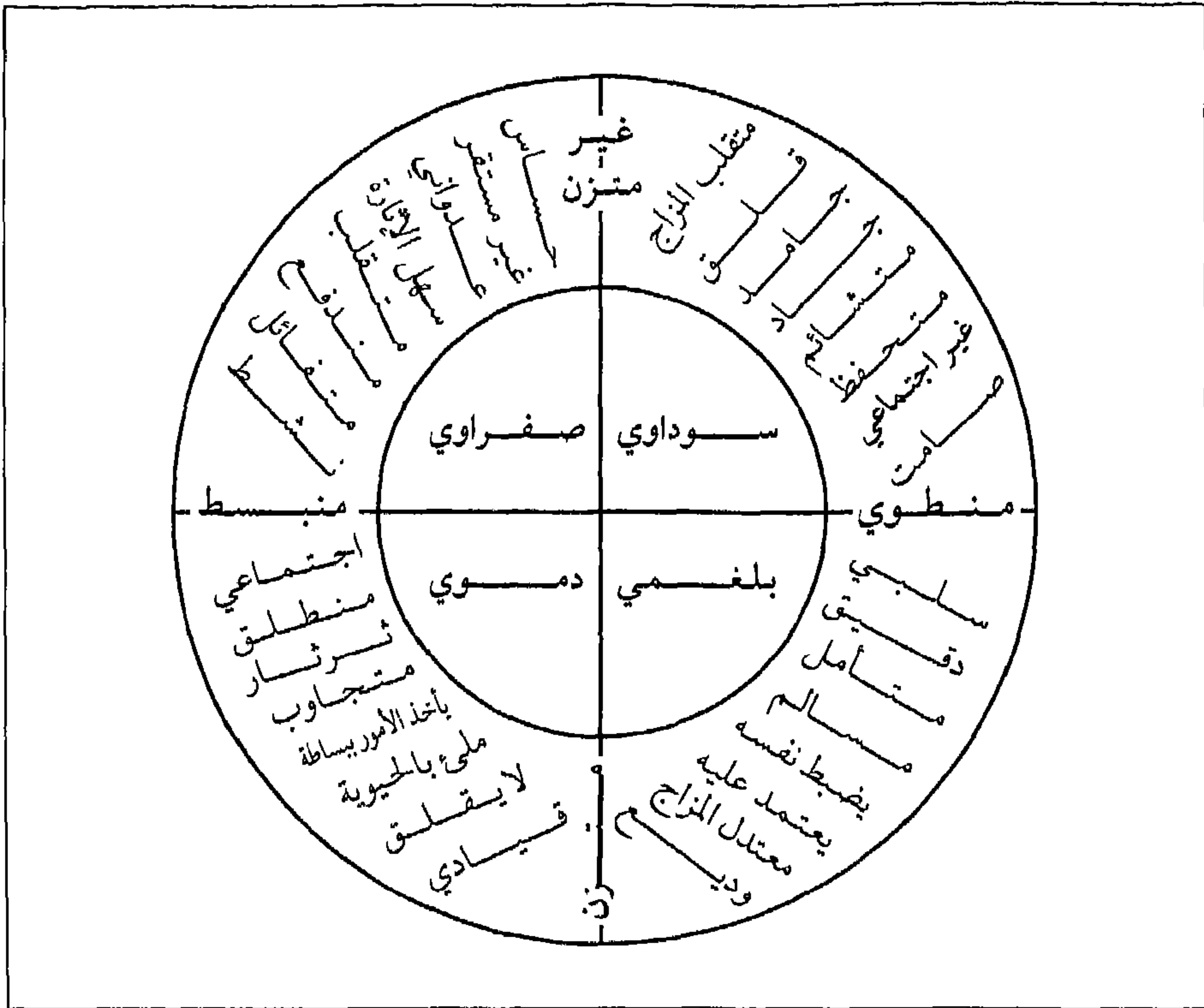
شكل (٥) : علاقة بعدي الانبساط والعصابية بنظريات الشخصية المبكرة
