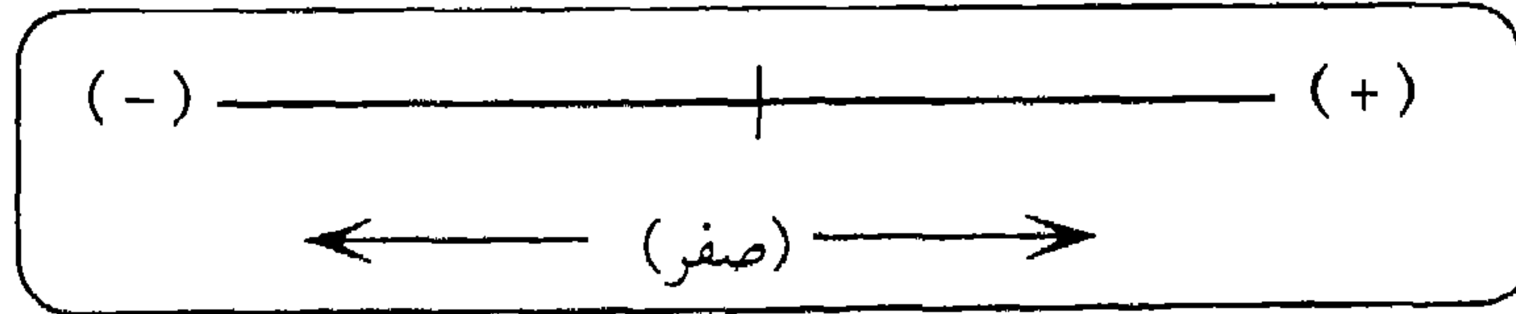
شكل (٢) : بعد (سمة) ثنائي القطب
