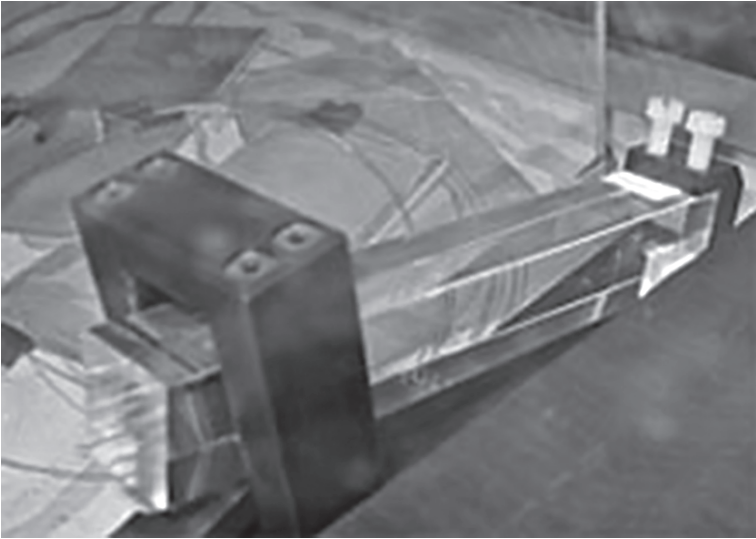
شكل ١٣-٨: صورة فوتوغرافية لبلورة تنجستات الرصاص المُستخدَمة في المُسرِّع الكهرومغناطيسي باللولب المركب للميونات.
