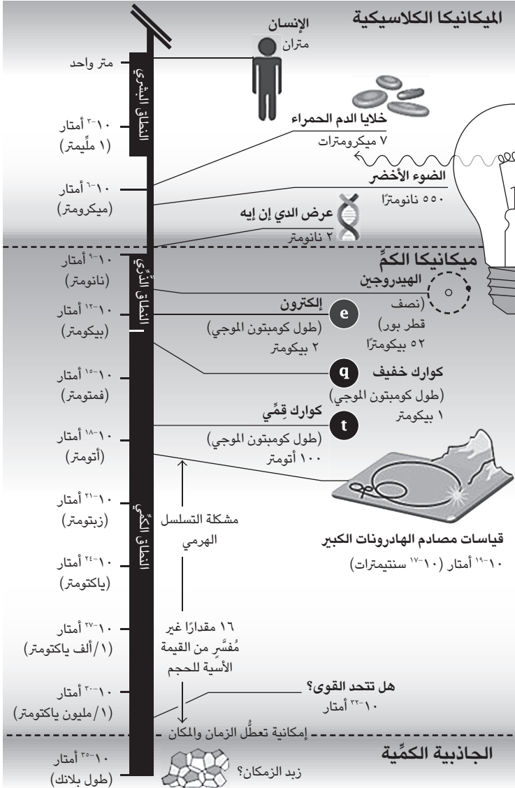
شكل 5-1: جولة في النطاقات الصغيرة ووحدة الطول المستخدمة في وصف هذه النطاقات.
