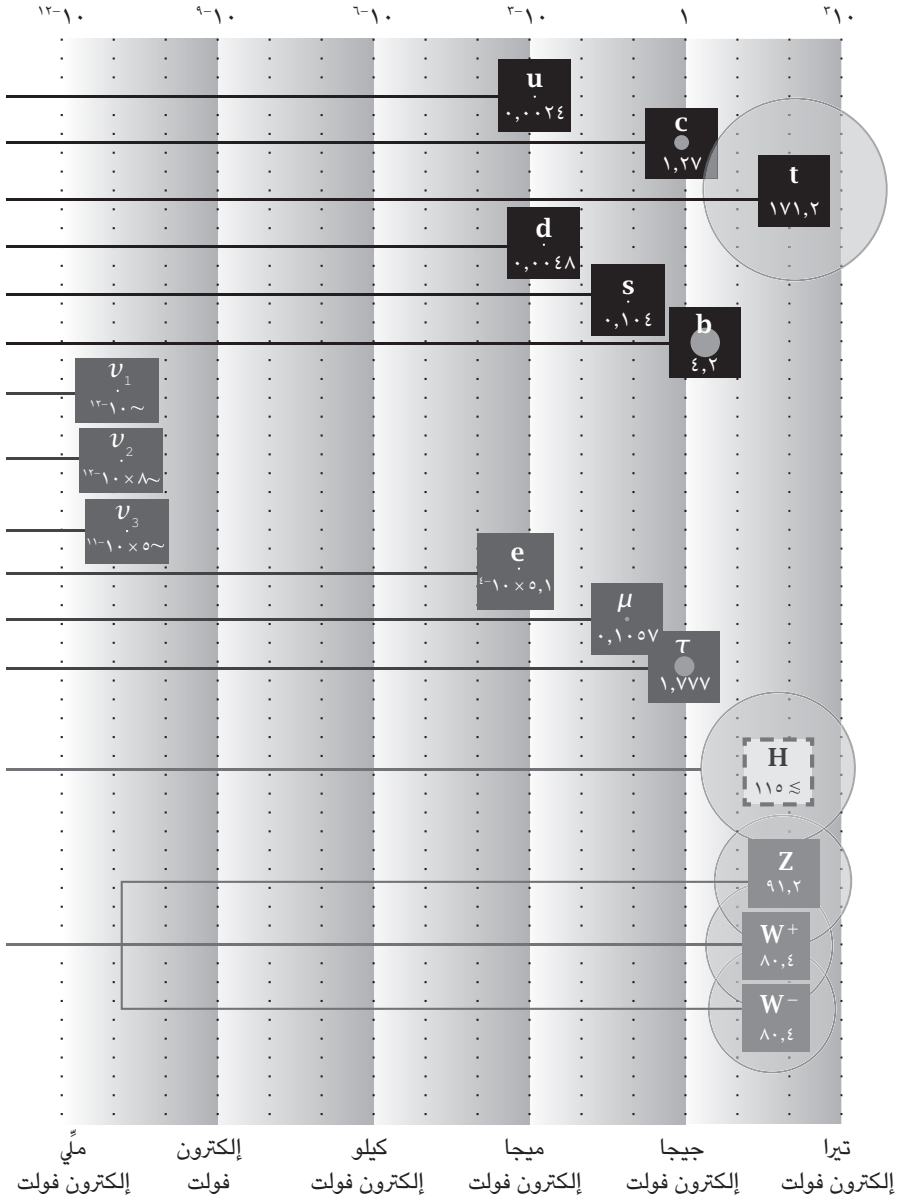
شكل ١٤-٧: ملخص لجسيمات النموذج القياسي مرتبّة حسب النوع والكتلة. والدوائر الرمادية (الموجودة أحياناً داخل المربعات) توضّح كتل الجسيمات. يتّضح لنا من هذا الشكل التنوّع الغامض لعناصر النموذج القياسي.
