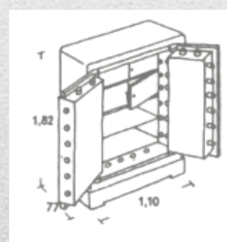
صورة توضح أبعاد خزانه
