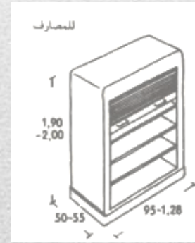
صورة توضح أبعاد خزانه للمستندات
