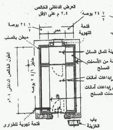
تفصيله المسقط الافقى للخزينة
