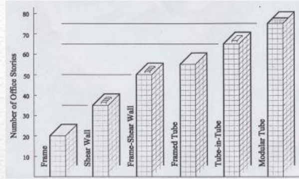
مخطط يوضح عدد الأدوار التي يمكن عملها من كل نظام إنشائي خرساني
