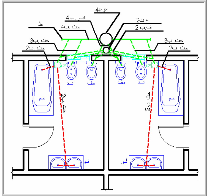
شكل رقم (44) - صرف الحمامات بنظام الماسورة الواحدة المهواة بالكامل
