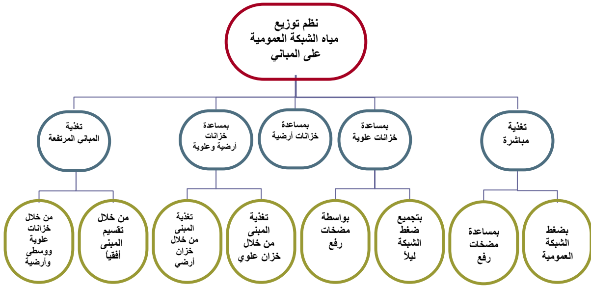
شكل رقم (50) - نظم توزيع مياه الشبكة العمومية على المباني
