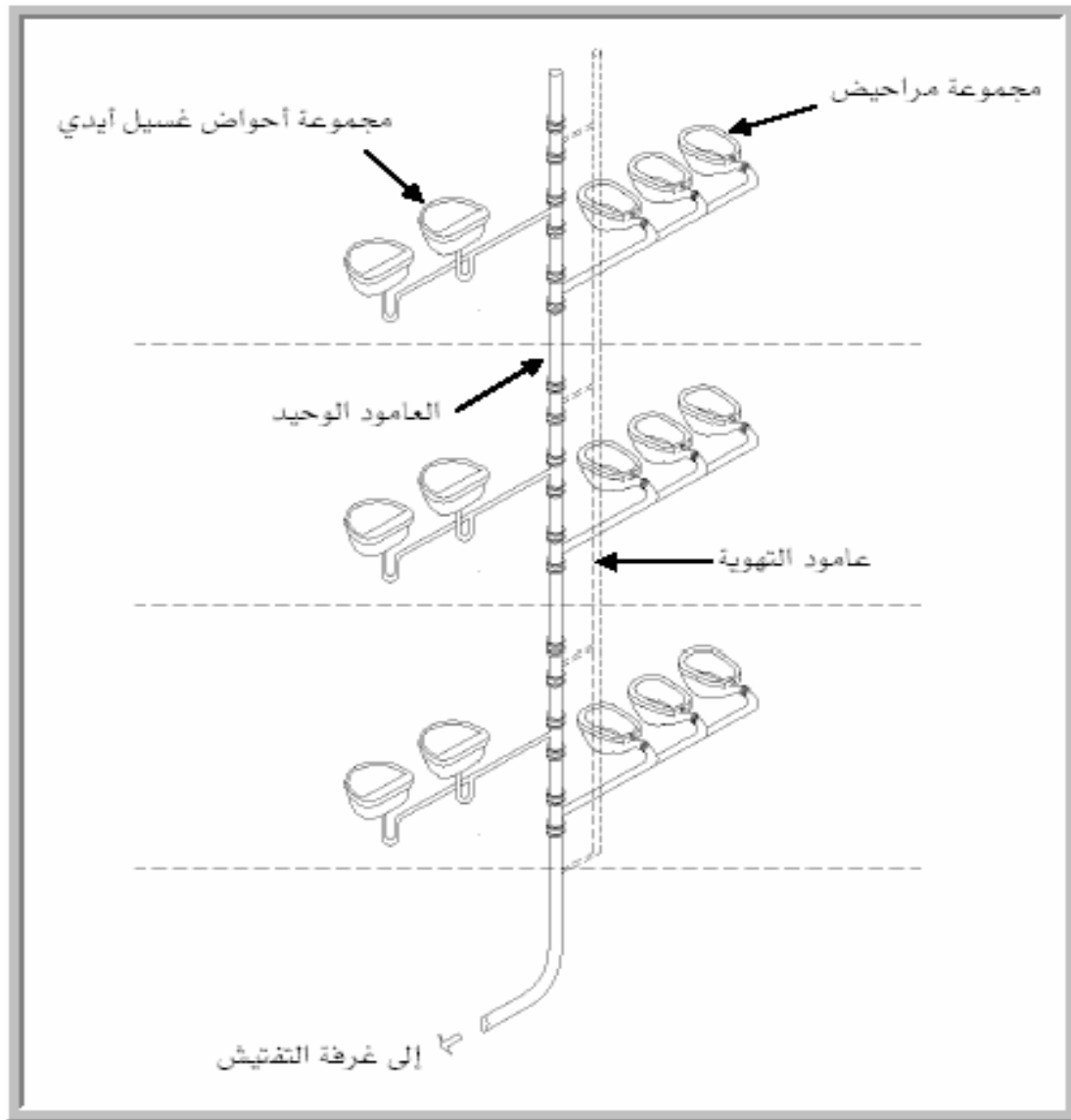
شكل رقم (38) - أسلوب العامود الوحيد مع عمود الهواء
