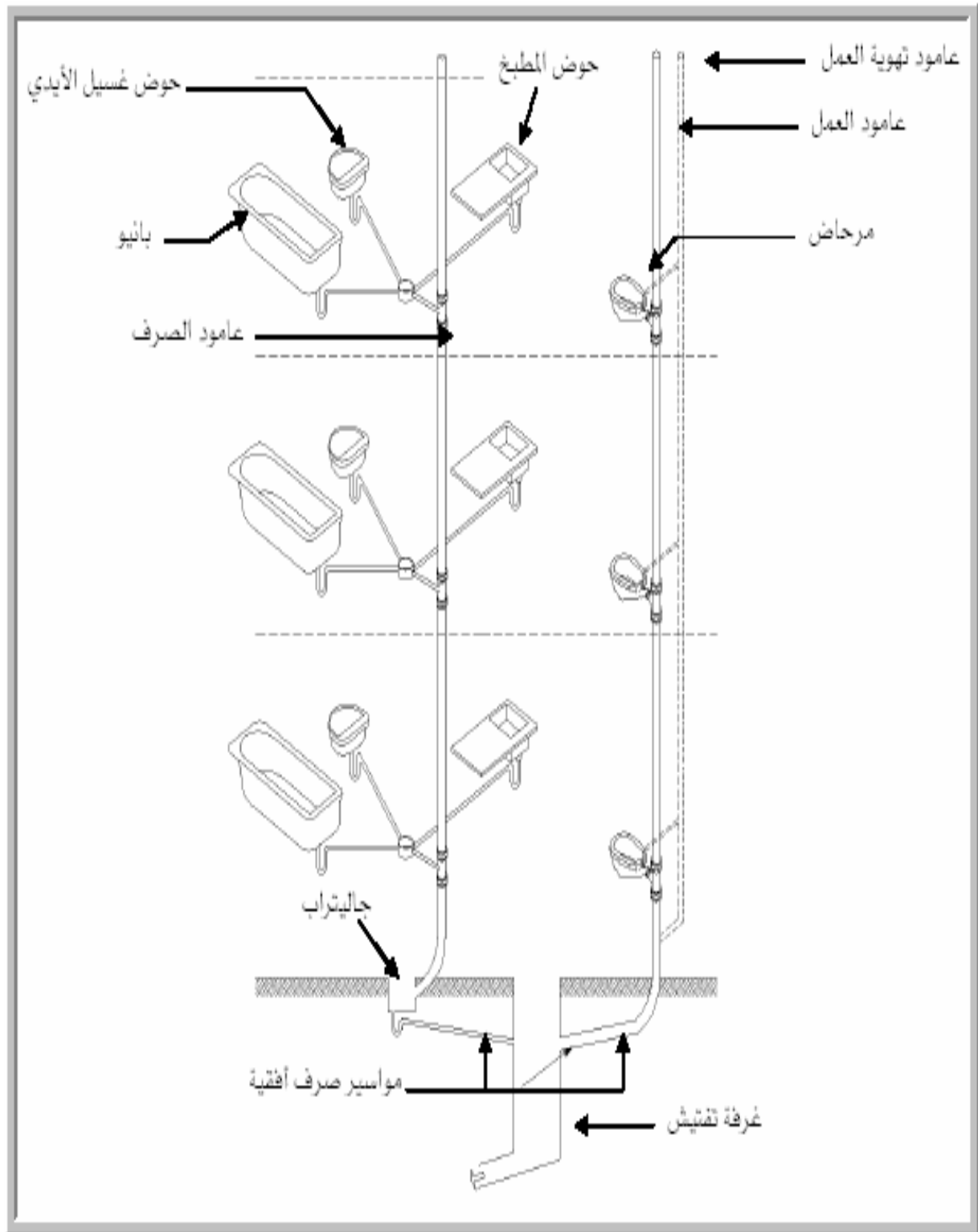
شكل رقم (33) - أسلوب الماسورتين بسيفون أرضي مع تهوية عمود العمل
