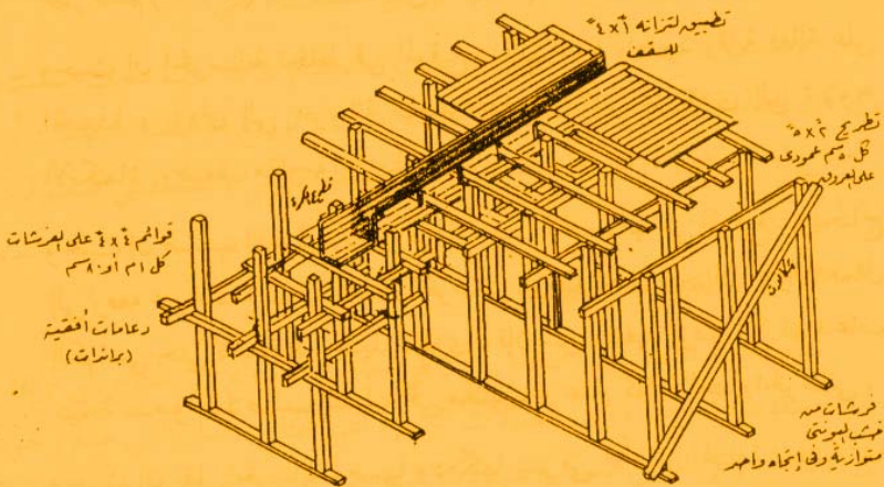
شادات الأسقف التقليدية
