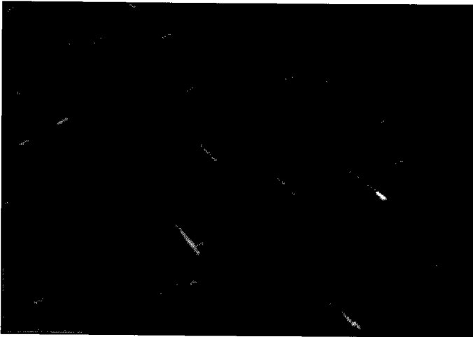
مجموعة من الشهب الساقطة والصورة توضح كثافتها. وللشهب أوقات في السنة تزداد أعدادها
