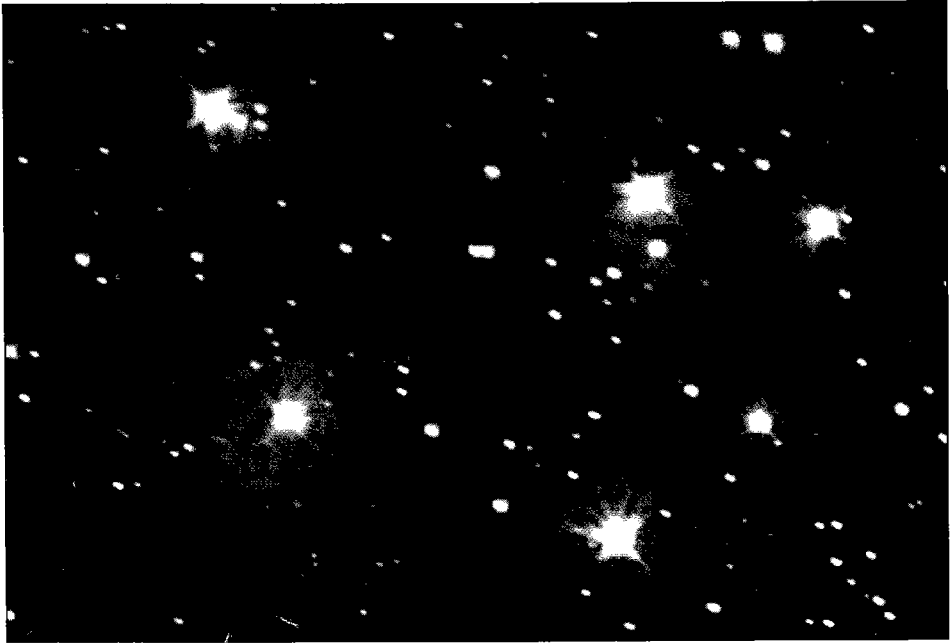
الشمس أو النجوم طاقات هائلة من الانصهار النووي تبدو قريبة في الصورة ولكن ما بينها آلاف الملايين من الكيلو مترات
