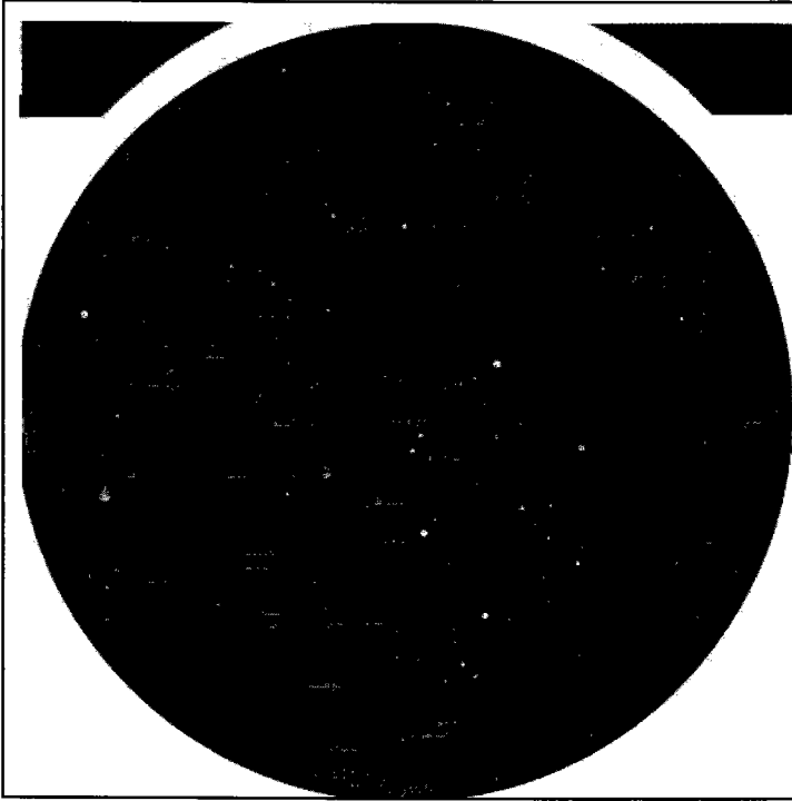
القبه السماوية ويظهر فيها النجوم المتبدلة - النجوم المزدوجة مجموعة العناقيد المفتوحة والكروية مجرات - سحبات سديمية كوكبية
