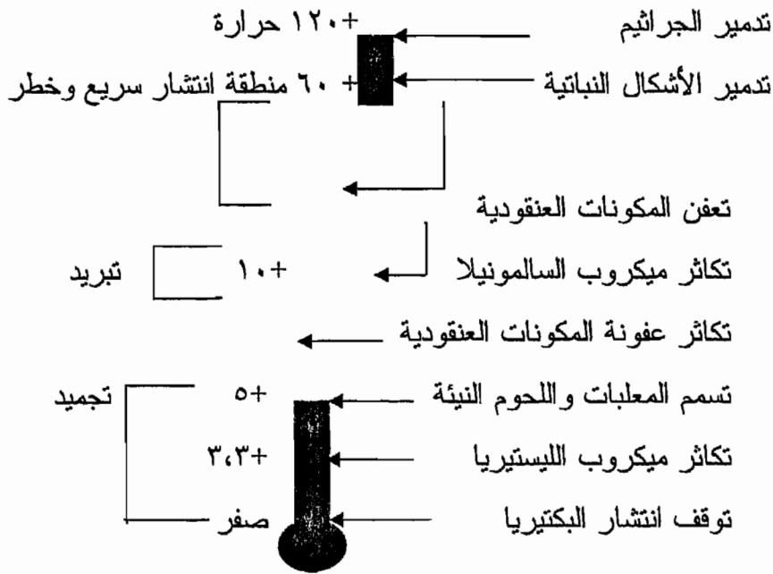
شكل (٢) دور الحرارة في نمو الجراثيم
