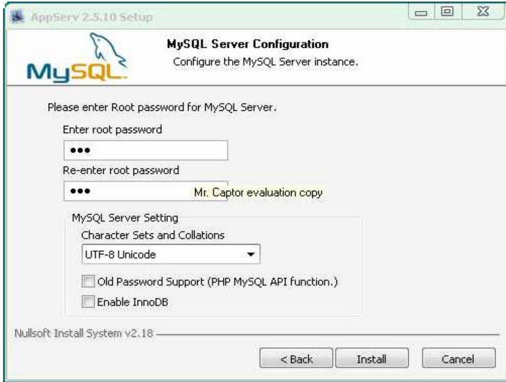
شكل (6) تحديد كلمة السر الخاصة بمدير قواعد البيانات
