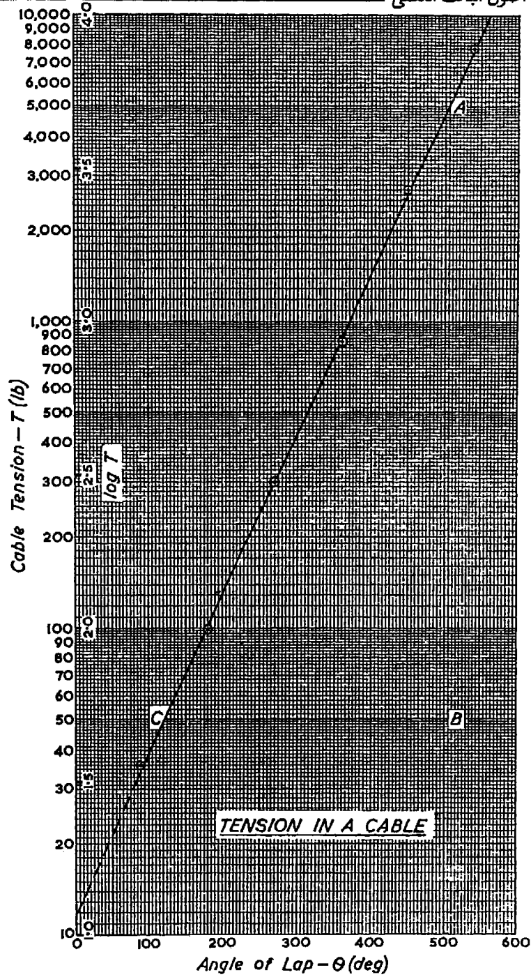
شكل ( ٥ - ٨ ) : رسم بياني ذو تدرج لوغاريتمي للمحور الرأسي . يلاحظ أن التغير غير المستقل يتراوح مداه بين ١٢ و ١٠٠٠٠ ، وأن العلاقة بين المتغيرين المستقل وغير المستقل أصبحت خطية بعد توقيع التغير غير المستقل على تدرج لوغاريتمي .
