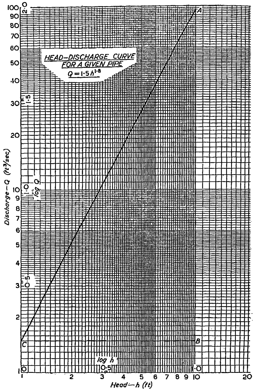
شكل ( ٥ - ٩ ) : رسم بياني ذو تدرج لوغاريتمي للمحورين الأفقي والرأسي . يلاحظ أن العلاقة بين المتغيرين أصبحت خطية بعد توقيعهما على تدرجات لوغاريتمية
