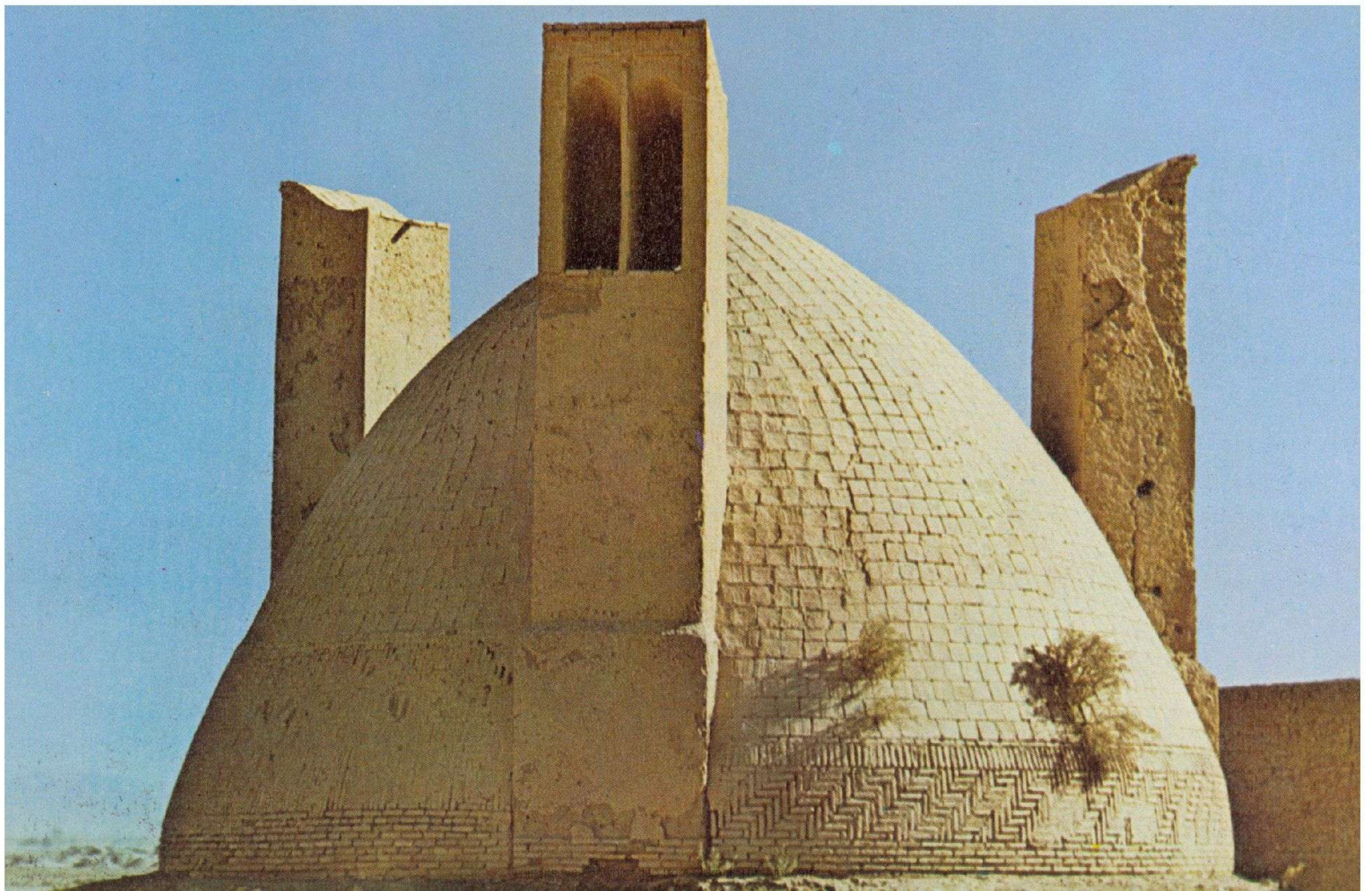
١٥٢ شكل يمثل الطريقة التقليدية لحفر بئر في المناطق الجافة ببلاد فارس . وعمارة هذا الصرح الضخم الواقع بين نائن ويزد تبين انه بمساعدة الريح التي تهوي الفضاء الداخلي يقل تكثف البخار الى ادنى حد ويظل الماء باردا سردا .
