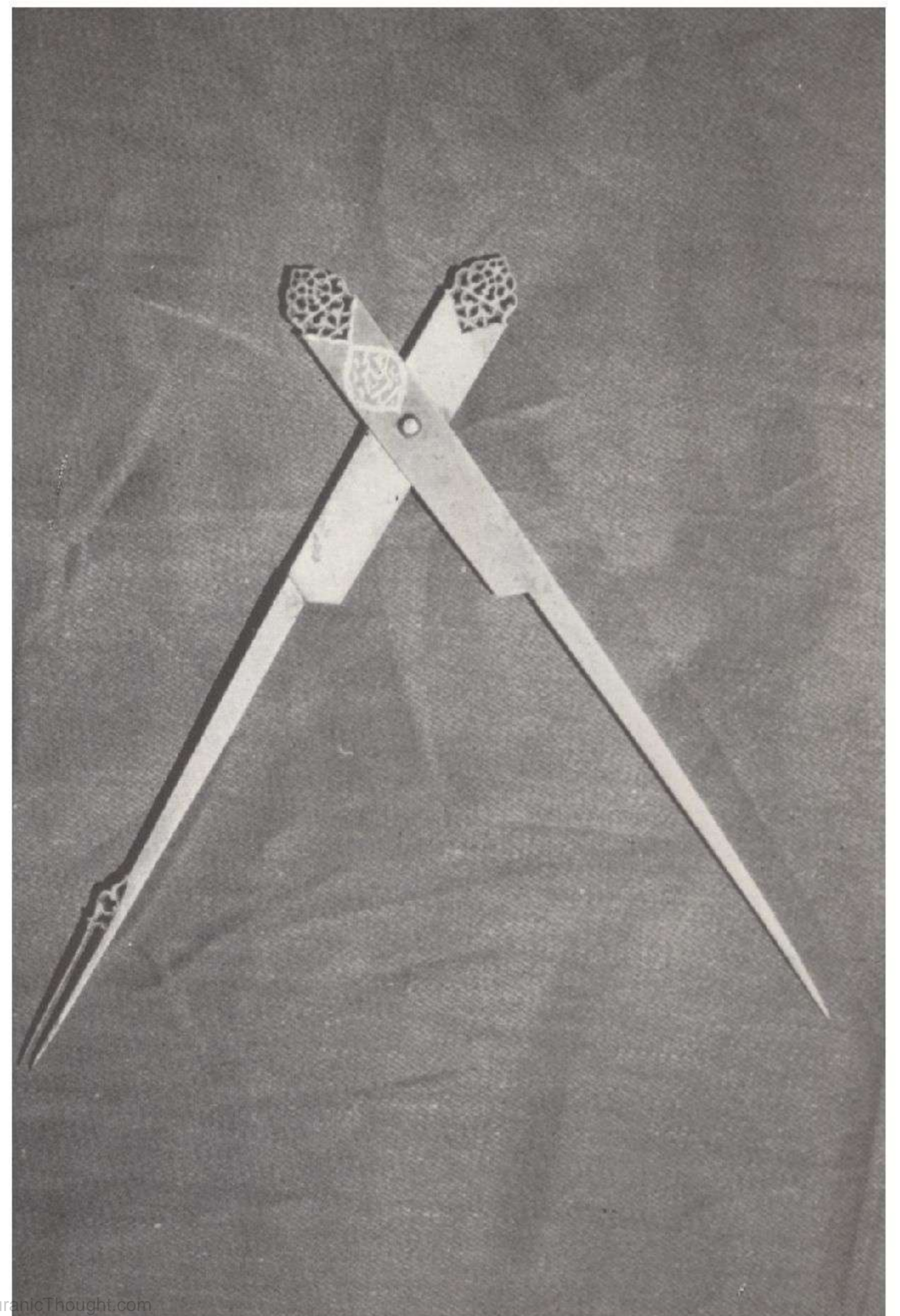
٤٥ هذا الشكل يمثل بوصلة من الصلب صنعت لملك فارسي شاه عباس .
