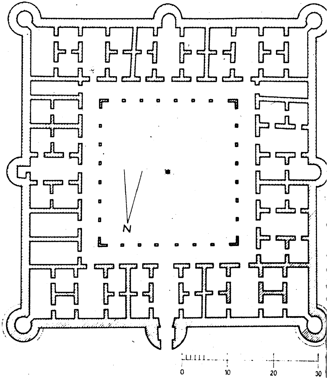
مخطط قصر اسييس في بادية الشام ٢ - مخطط قصر قصر عمره
